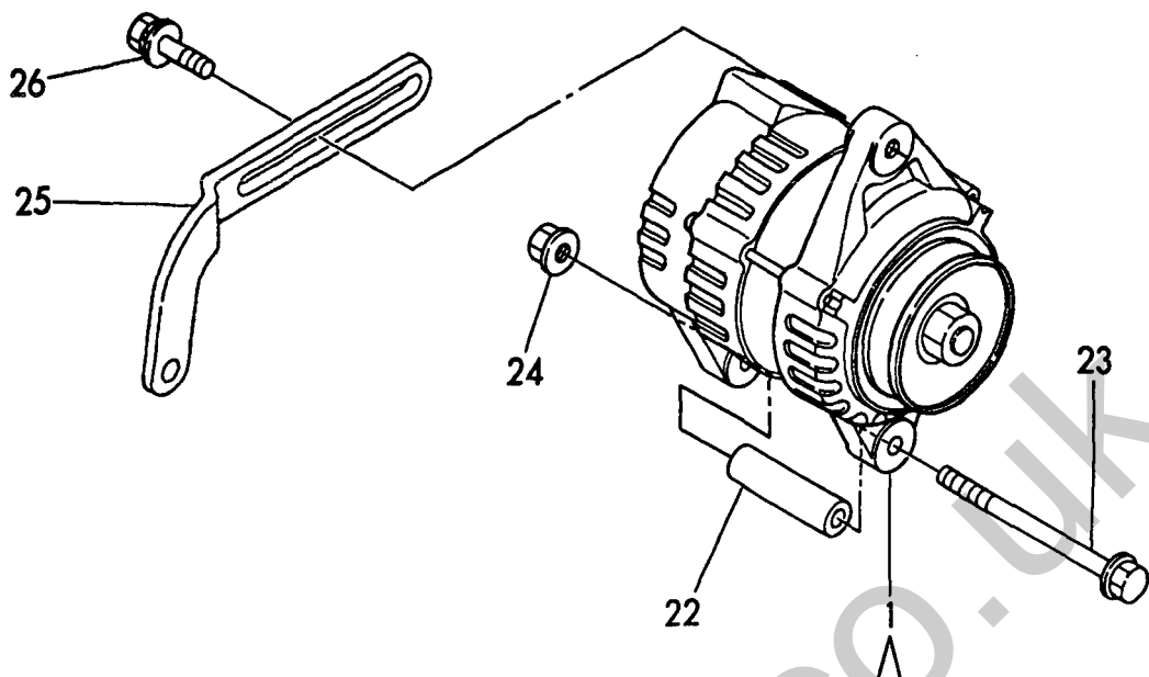
Fig. 18 GENERATOR
